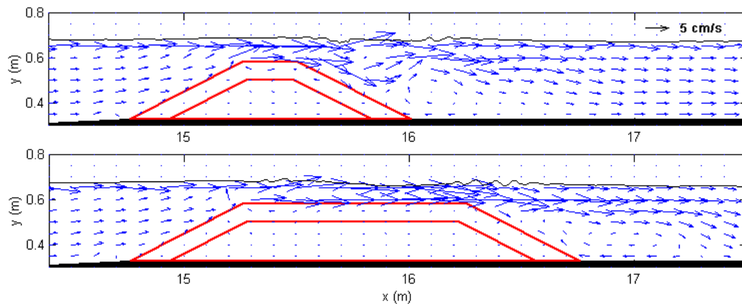
Figure 5. Champ des vitesses moyennes calculé par le modèle pour deux valeurs de la largeur de crête : 25 et 100 cm.
