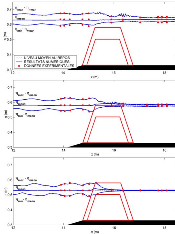
Figure 4. Enveloppes de hauteur de vague et niveau moyen pour trois valeurs de la profondeur d'eau au large : 0.40, 0.35 et 0.30 m.
