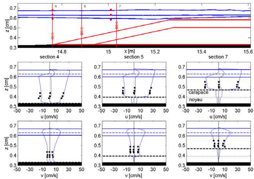
Figure 3. Profils verticaux des vitesses horizontales ( u ) et verticales ( v ). Profondeur d'eau au large = 0.40 m ; hauteur de houle = 0.07 m ; période = 1.6 s. Lignes continues : résultats numériques, points : données expérimentales.
