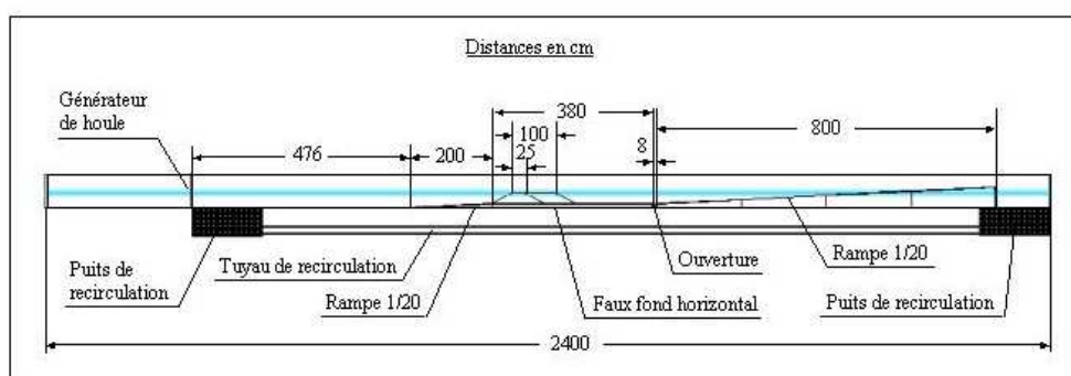
Figure 1. Configuration des essais.
