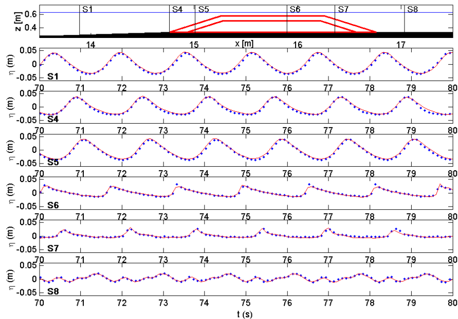
Figure 2. Séries temporelles de déplacement de la surface libre. Profondeur d'eau au large = 0.40 m ; hauteur de houle = 0.07 m ; période = 1.6 s. Lignes continues : résultats numériques, lignes en pointillé : mesures.
